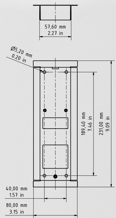
Montagerückgehäuse
